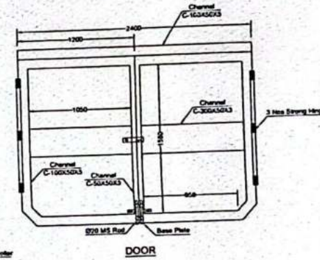
DOOR
